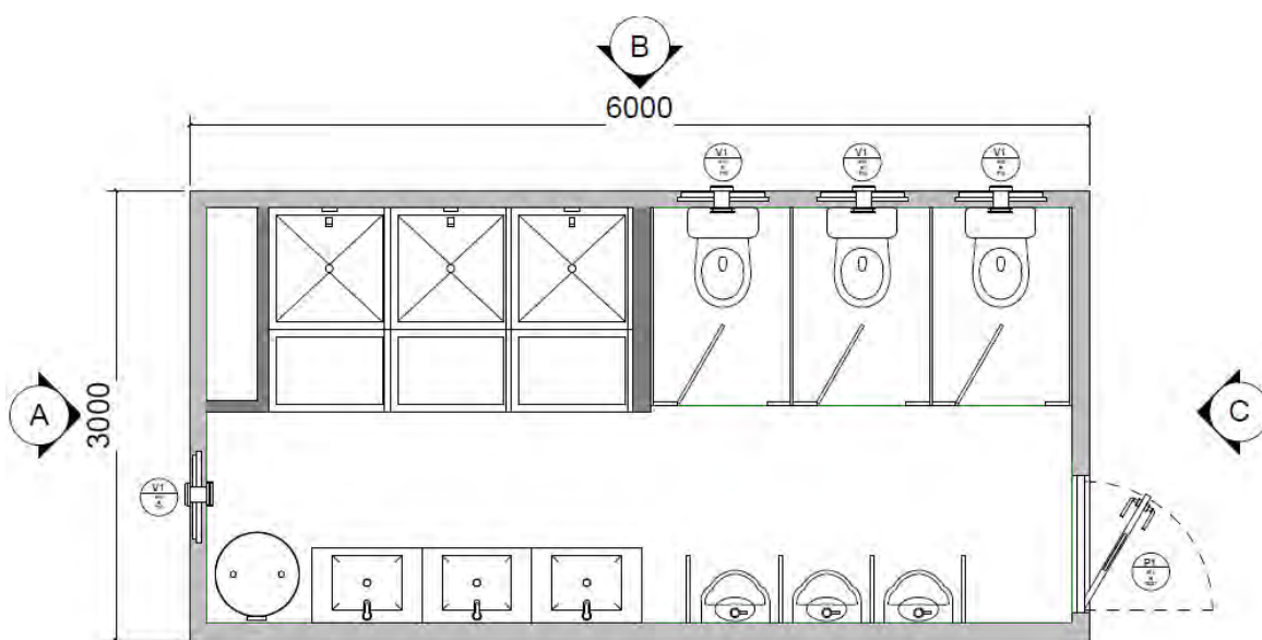
PLANTA DE ARQUITECTURA Esc: 1:25
