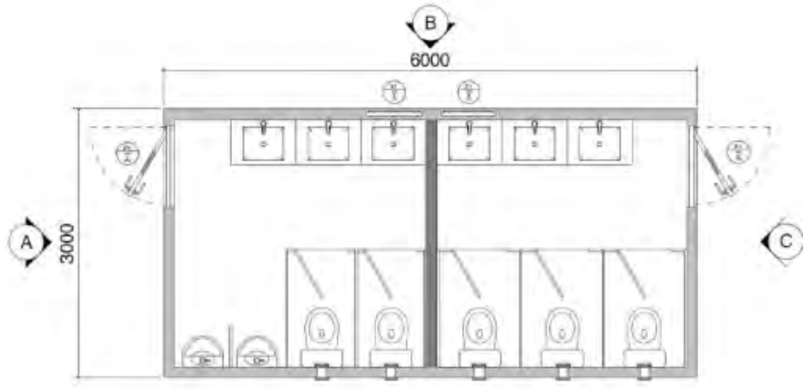
PLANTA DE ARQUITECTURA Esc 1 : 25 MODULO 18m2 D
