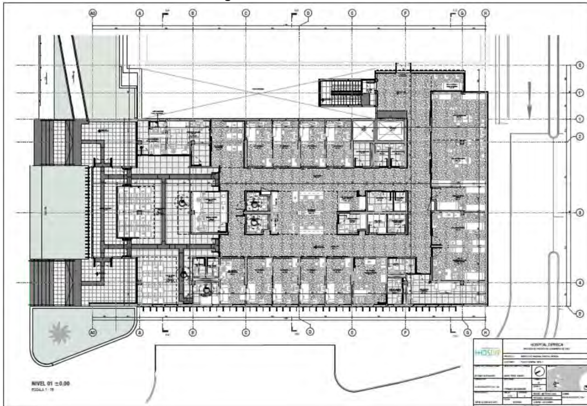
Figura N° 2.3: Planta Nivel1
