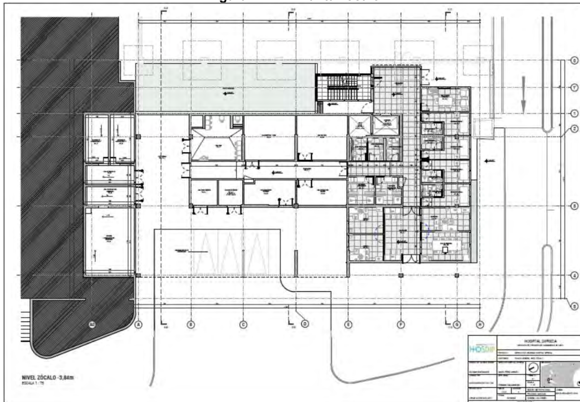
Figura N° 2.2: Planta zócalo
