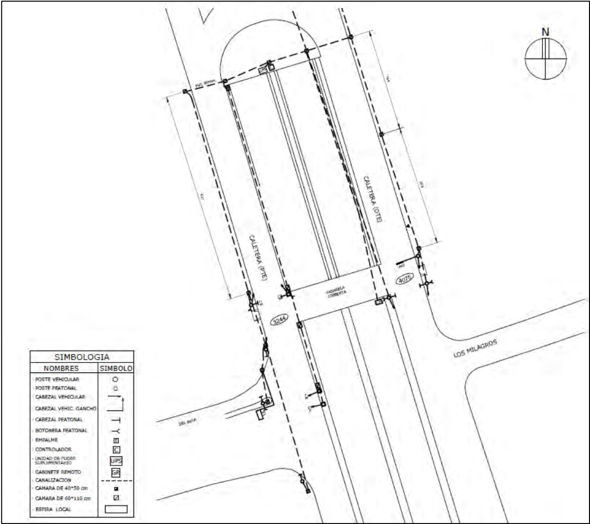
Figura N° 6-5 Catastro Cruce MANQUEHUE - DEL INCA - LOS MILAGROS (3244 / 4075)
