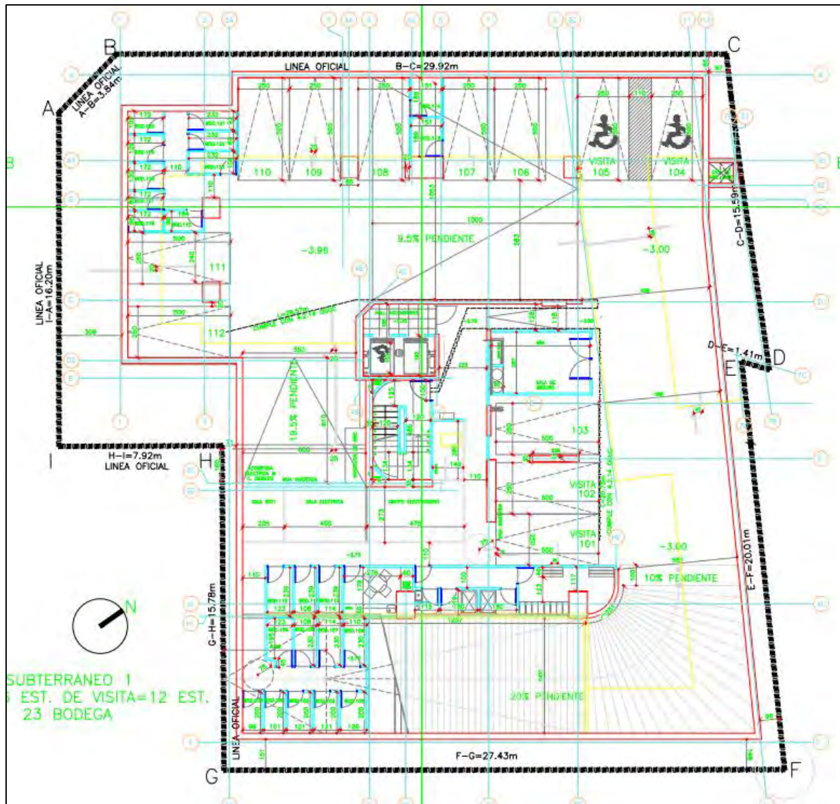
Figura N° 3.9: Subterráneo -1
