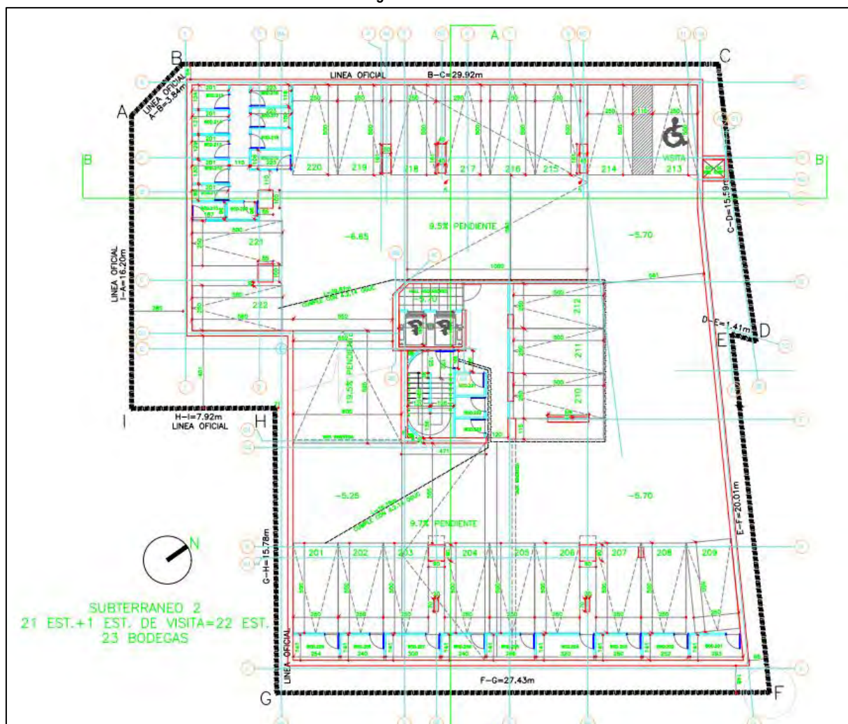
Figura N° 3.10: Subterráneo -2
