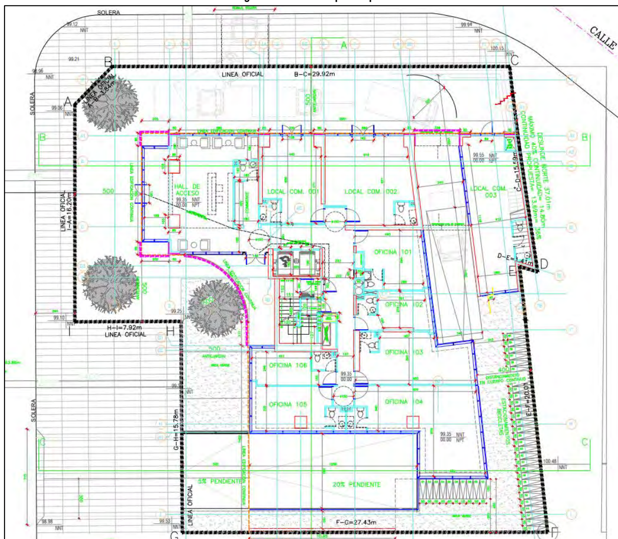
Figura N° 3.3: Planta primer piso
