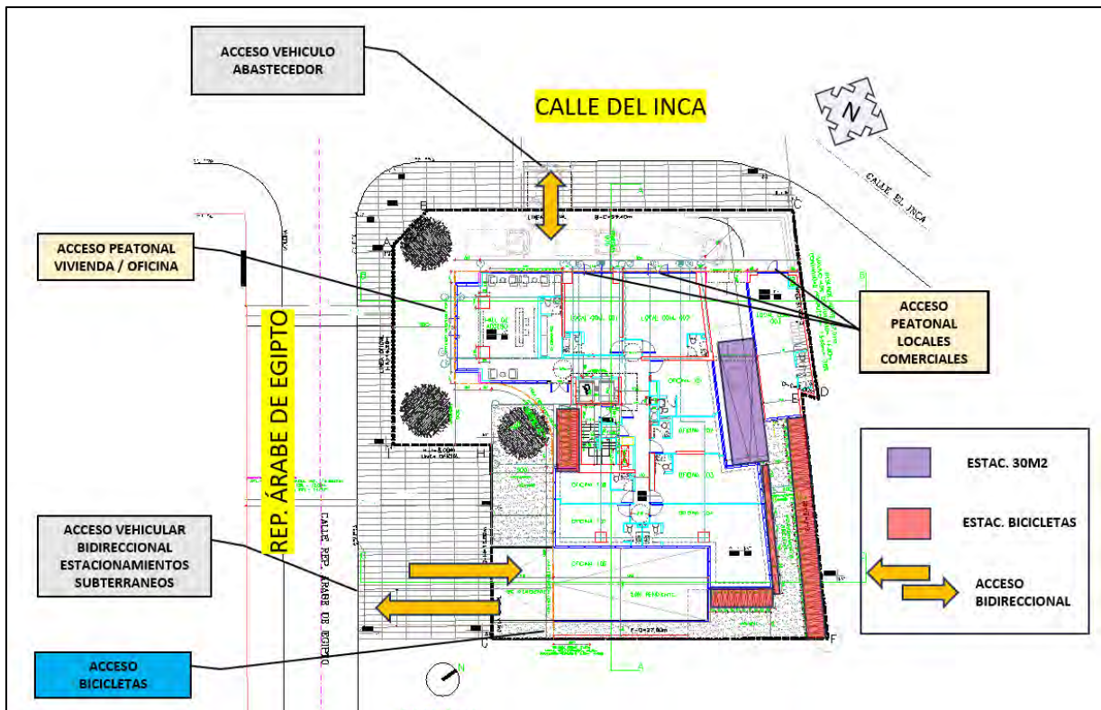
Figura N° 3.12: Emplazamiento - Detalle Acceso Peonatal y Vehicular
