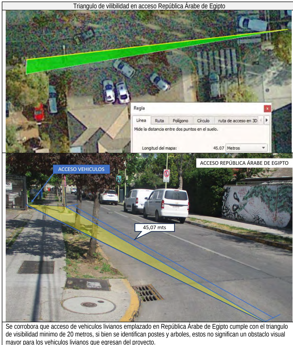
Figura N° 6-8 Triangulo de Visibilidad en Acceso República Árabe de Egipto.
