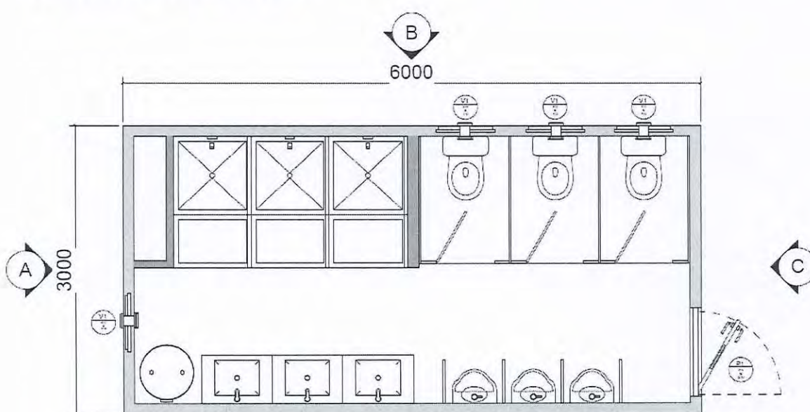
PLANTA DE ARQUITECTURA MODULO 18m 2 Esc. 1:25
