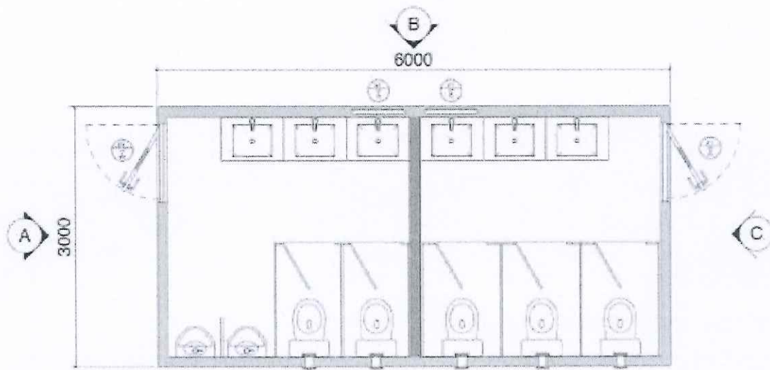
PLANTA DE ARQUITECTURA Esc 1:25 MODULO 18m2
