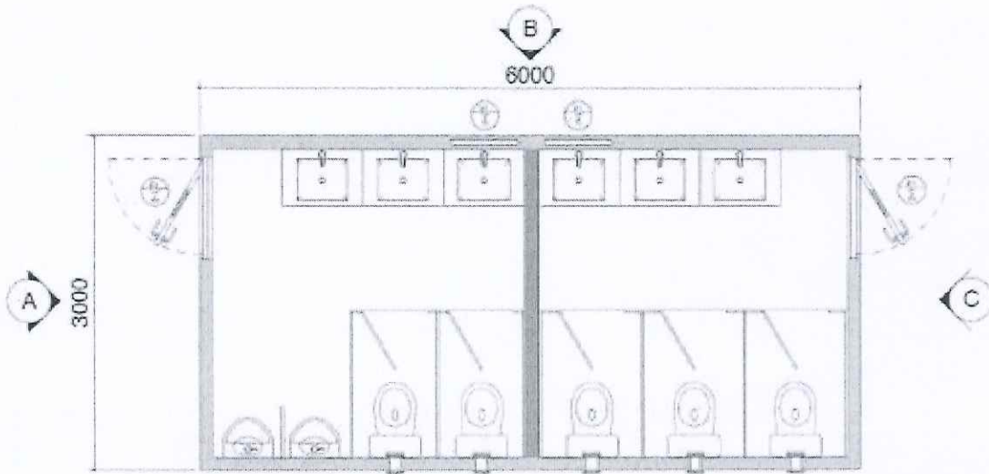
PLANTA DE ARQUITECTURA Esc 1 : 25 MODULO 18m2 D
