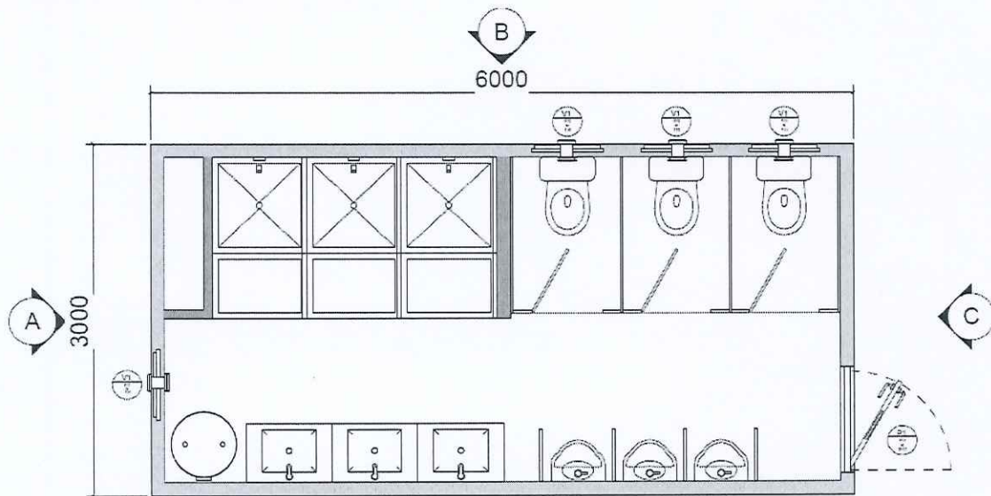
PLANTA DE ARQUITECTURA MODULO 18m 2
