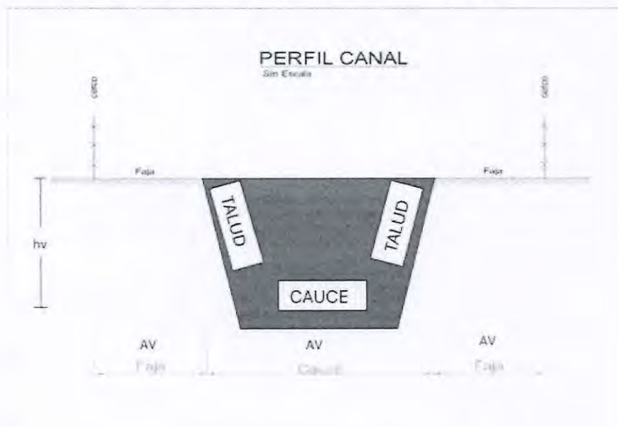
Imagen Referencial Perfil canal (Simbología: AV= Ancho variable; hv= Altura variable)
